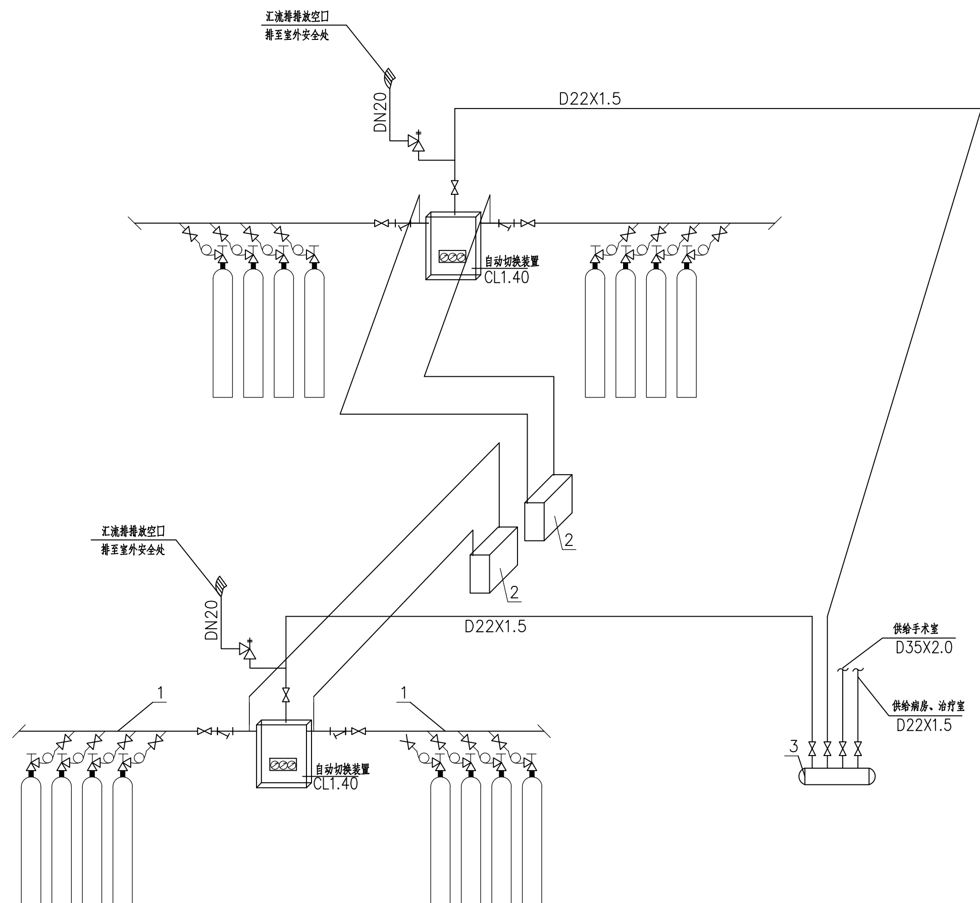
氧气汇流排工艺流程图
